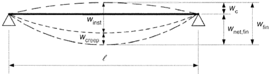
Fig. 3.8. Components of deflection (EN 1995-1-1).
