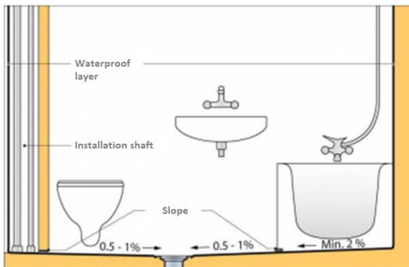
Fig. 3.48. Bathroom installations (SBI 252 Vådtrum).
