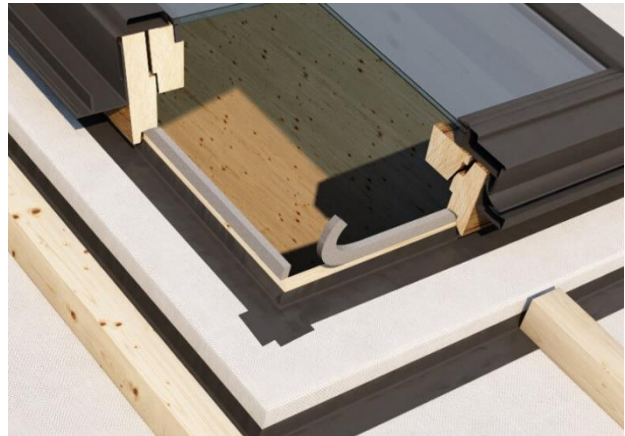
Fig. 3.33. Kompri band (Rothoblaas, 2020).
