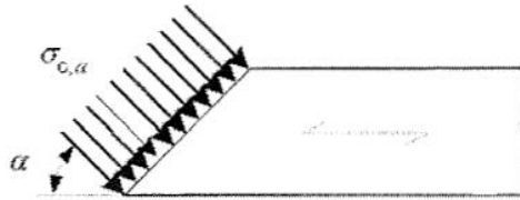
Fig. 4.7. Compressive stresses at an angle to the grain (EN 1995-1-1).
