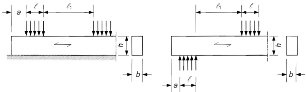
Fig. 3.5. Application of loading perpendicular to the grain (EN 1995-1-1).
